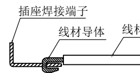
焊接 (钩焊) 示意图
