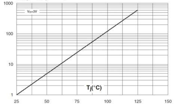
I_R(T_J) / I_R(T_J=25^{\circ}C)
