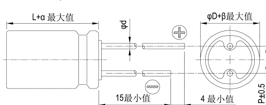
8φ×11.5L与10φ×12L
