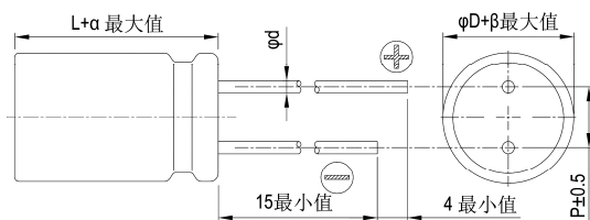
6.3φ与8φ×8L
