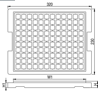
盘式包装
