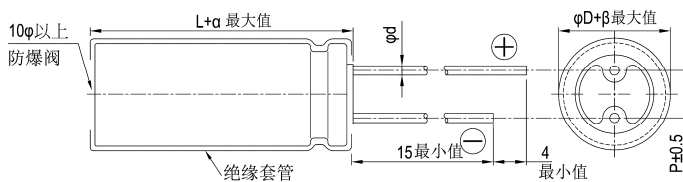
寸法图
