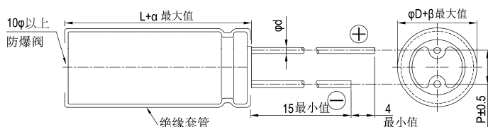
寸法图
