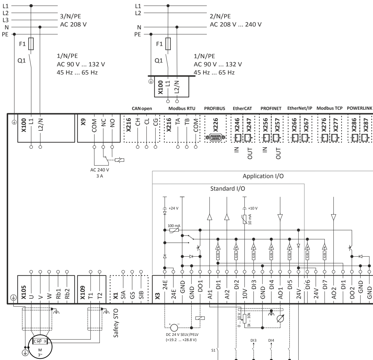
Fig. 3: Wiring example
