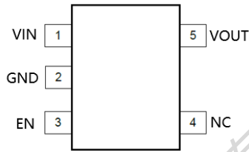
SOT23-5A
