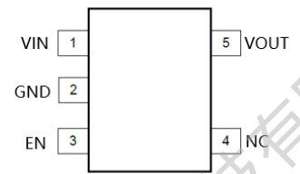
SOT23-5L
