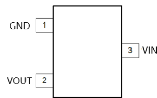
SOT23/SOT23-3L
