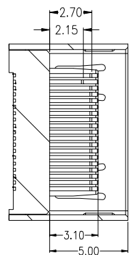
SECTION A-A
