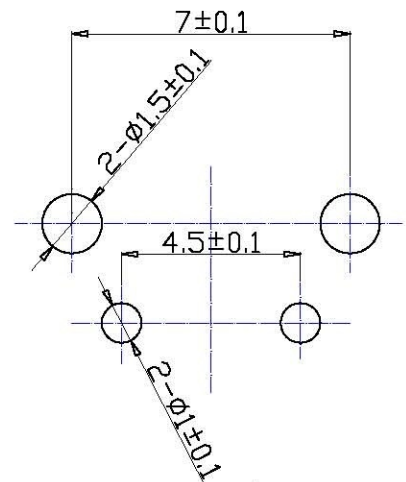
P. C. B. Land Pattern
