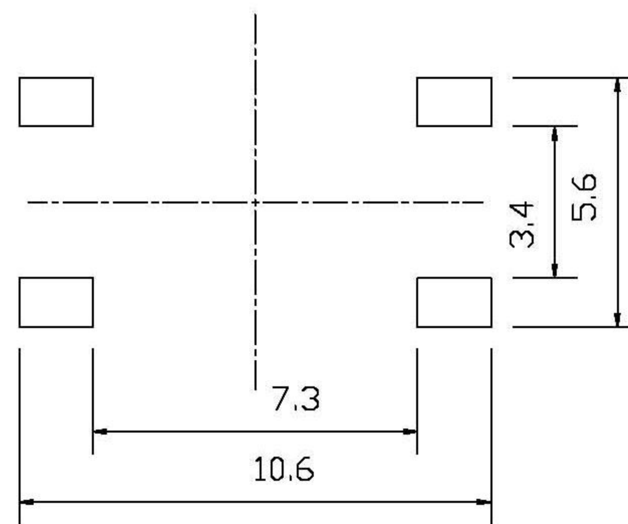
印刷线路板(PCB Layout)
