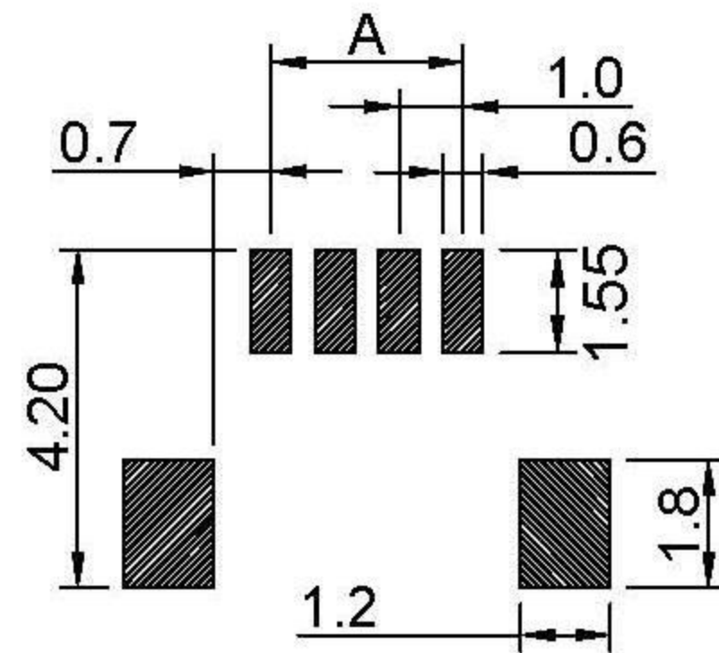
P.C.B LAYOUT
