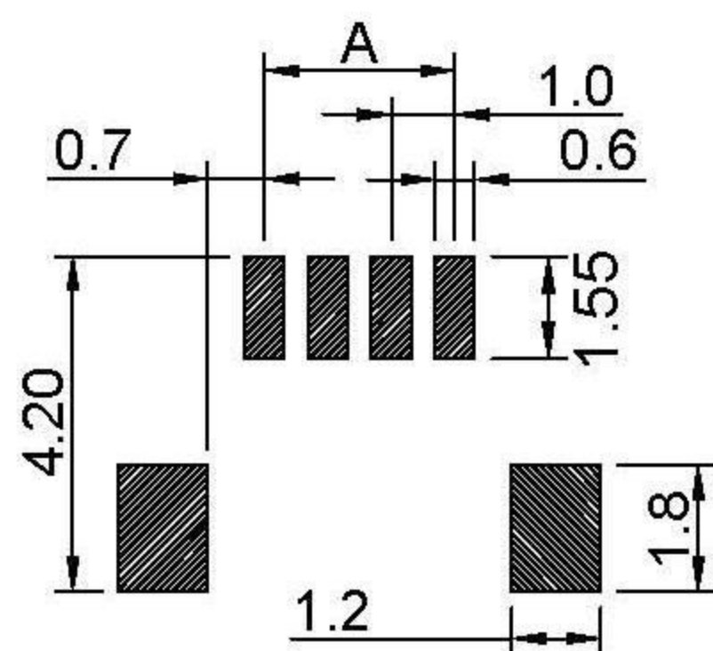
P.C.B LAYOUT
