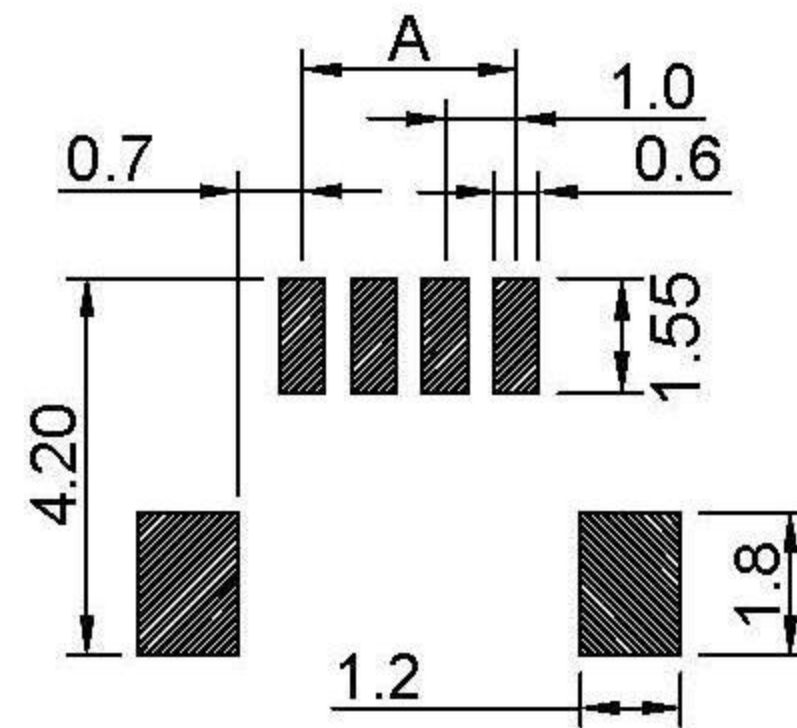
P.C.B LAYOUT
