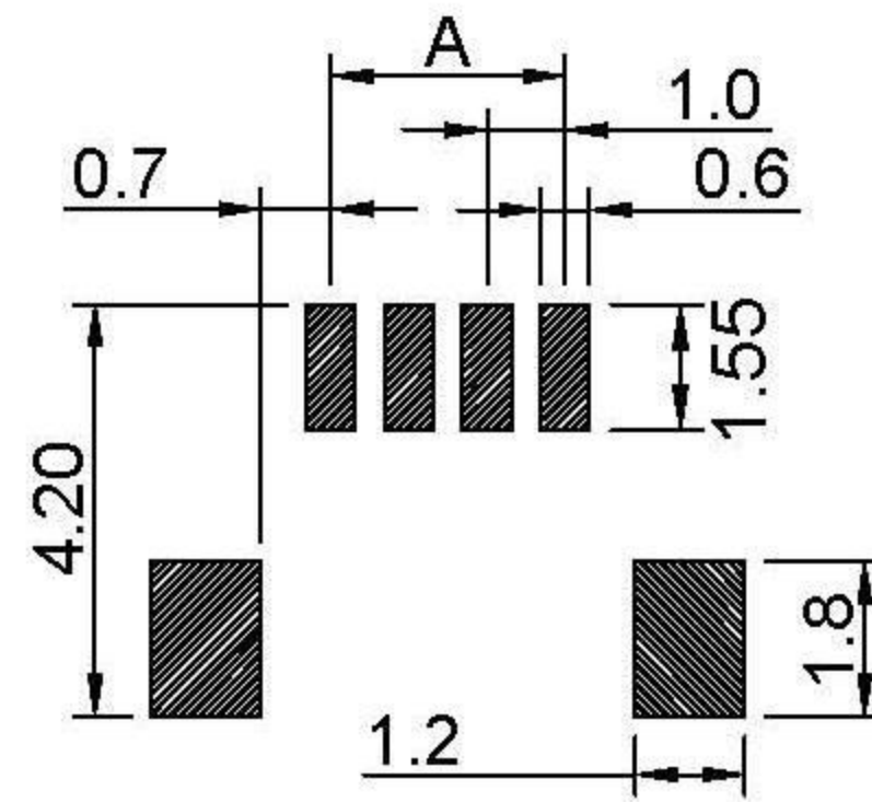
P.C.B LAYOUT
