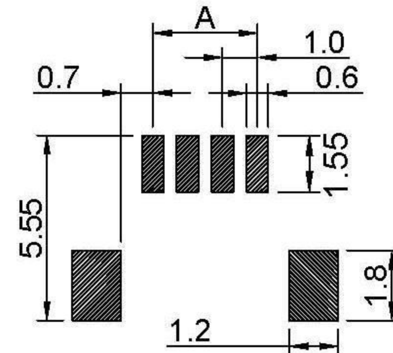
P.C.B LAYOUT
