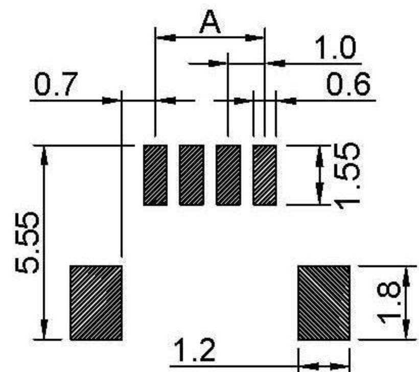
P.C.B LAYOUT
