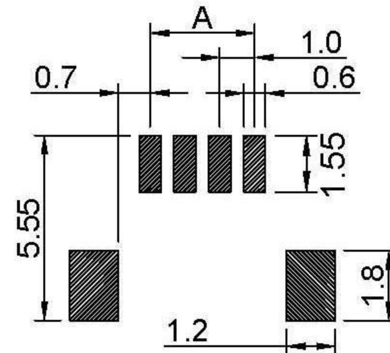
P.C.B LAYOUT
