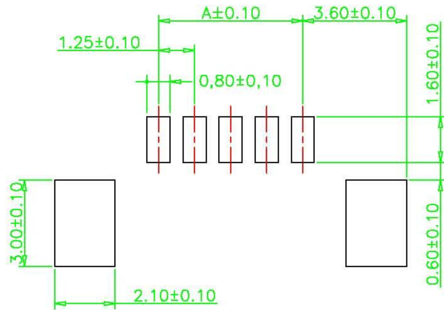
P.C.B LAYOUT
