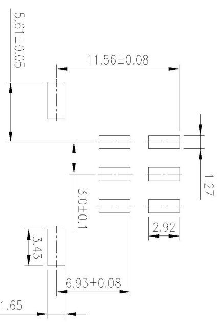
P.C.B LAYOUT
