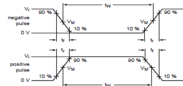
a. Input waveform
