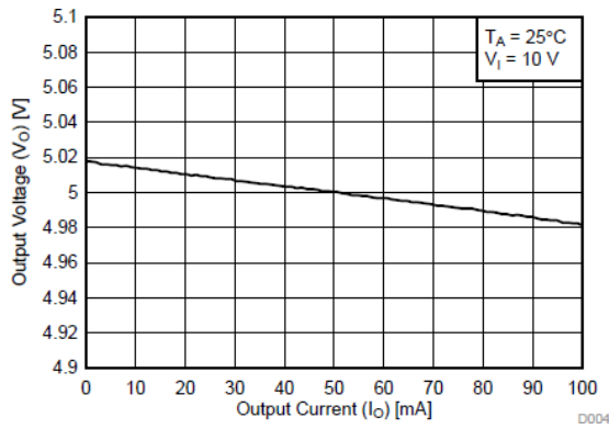
负载调整率
