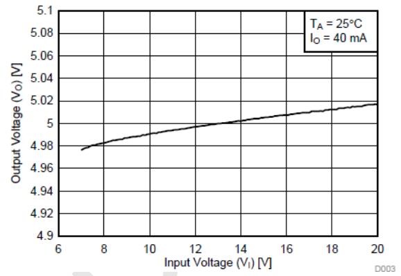
线性调整率
