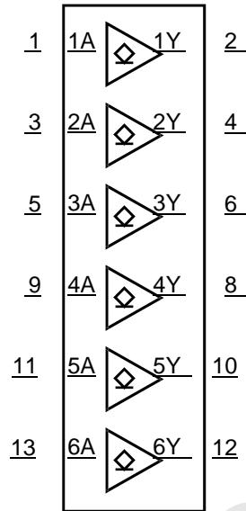
图1 逻辑符号
