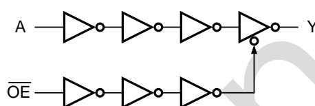
图 3 逻辑框图
