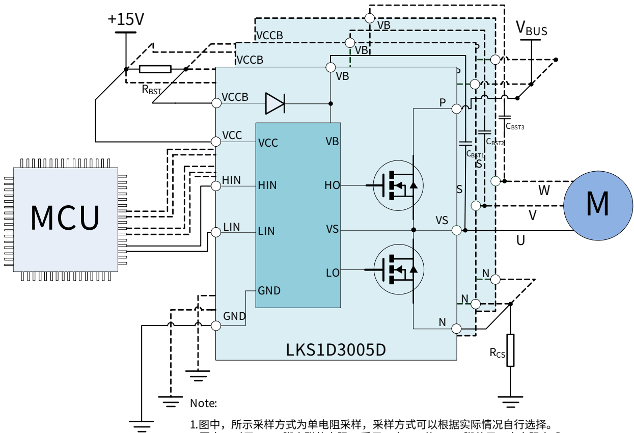
图 1. LKS1D3005D 典型应用图
