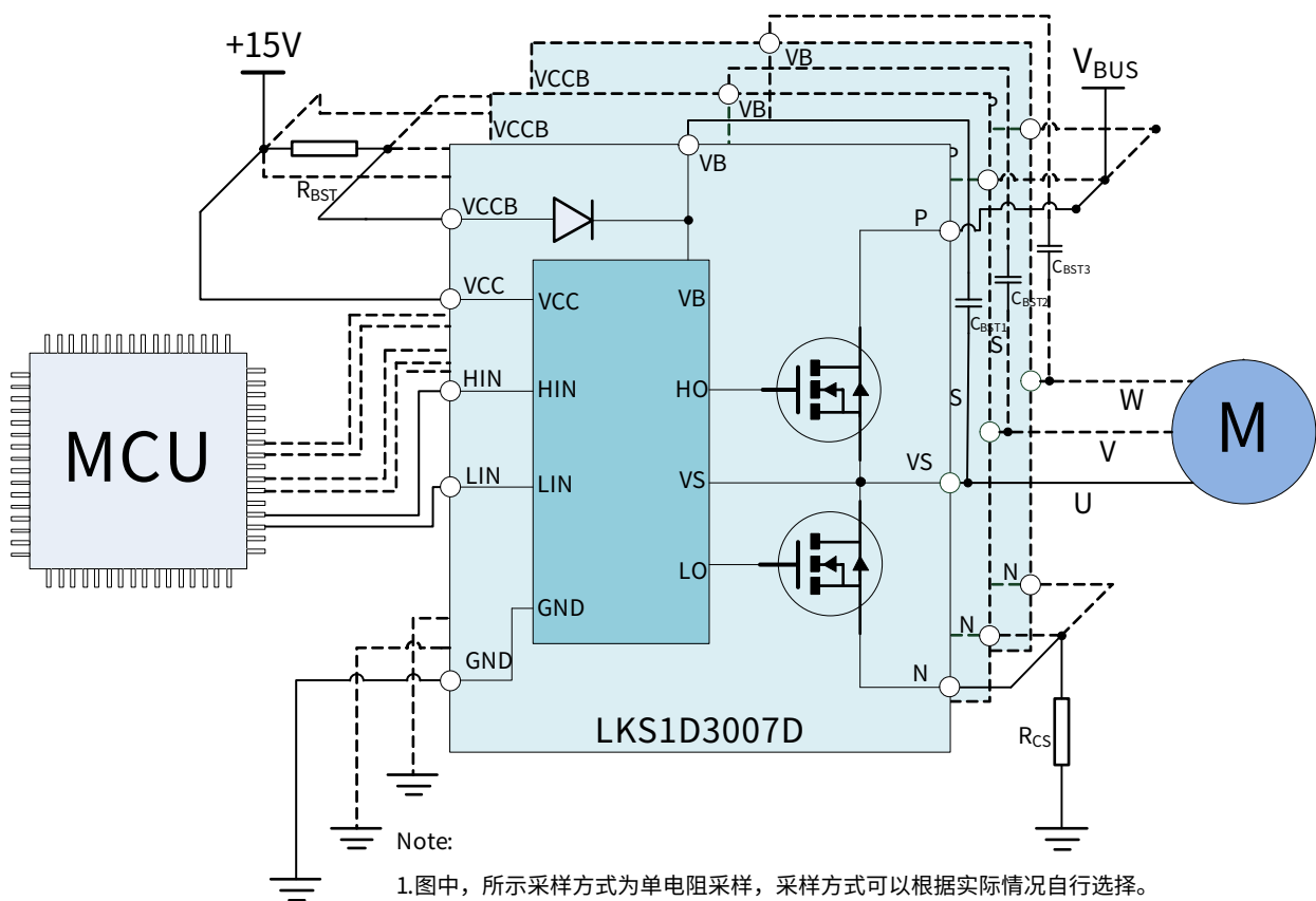
图 1. LKS1D3007D 典型应用图
