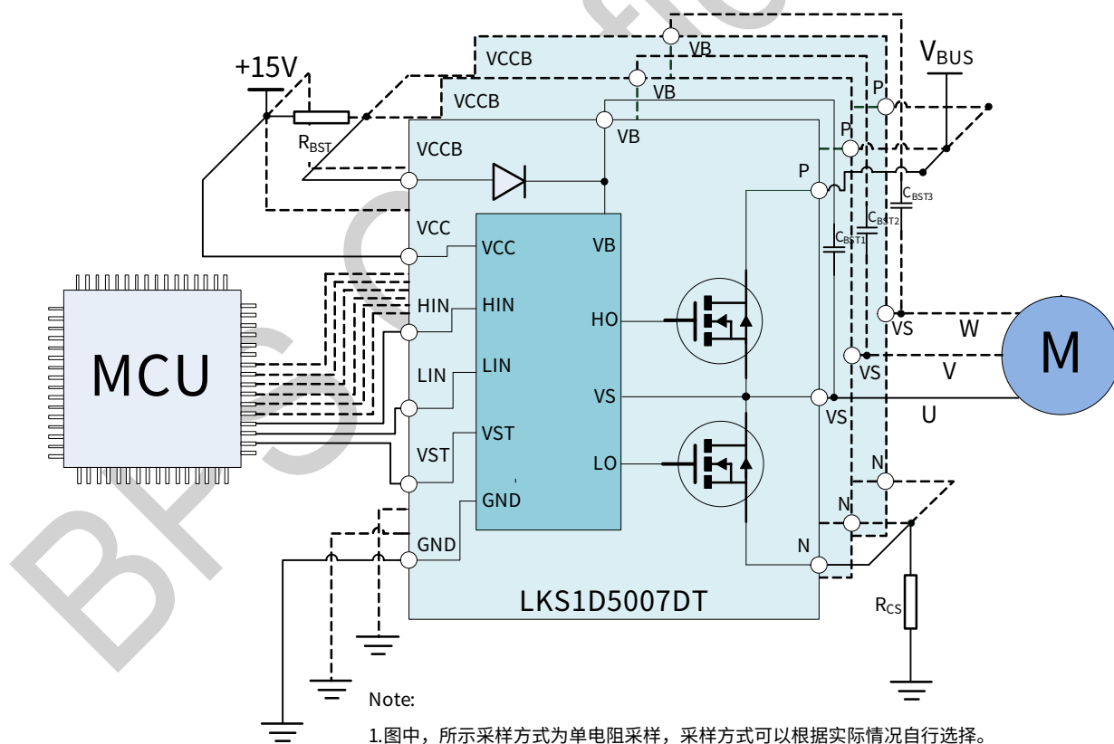
图 1. LKS1D5007DT 典型应用图
