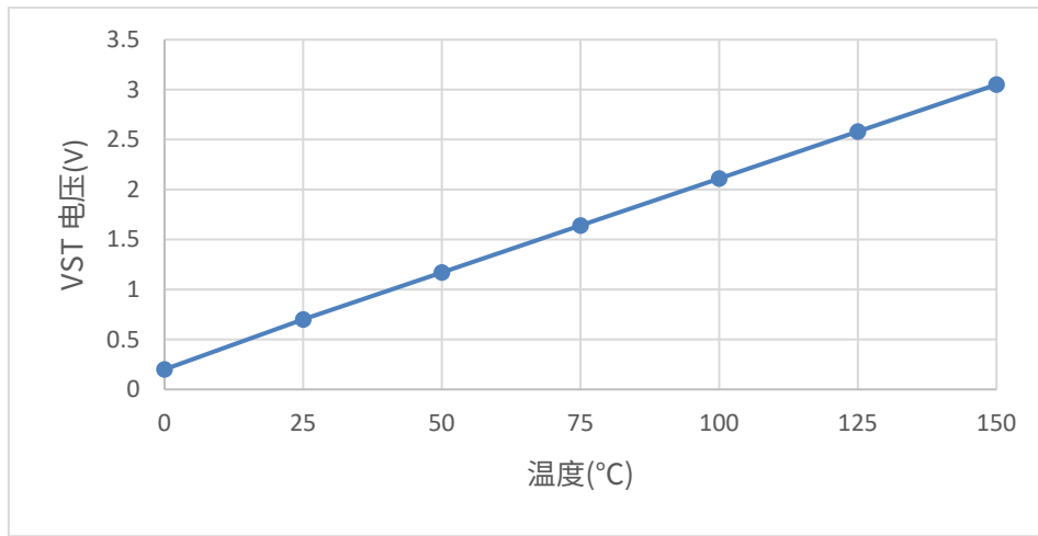
图 4.VST 输出特性曲线
