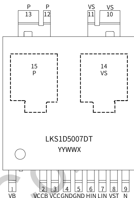
图 2. LKS1D5007DT 管脚封装图
