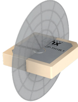
YZ-Plane Gain
