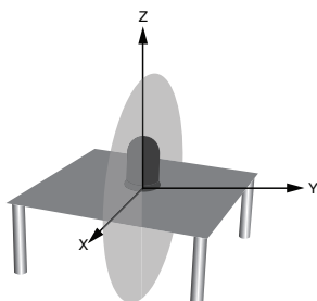
XZ-Plane Gain
