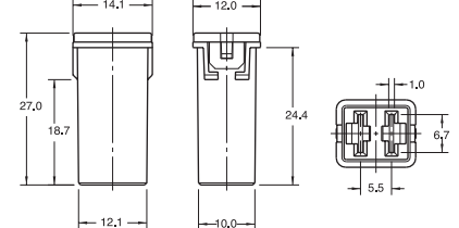
Dimensions JCASE®
