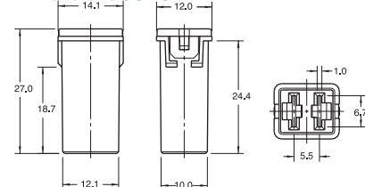
Dimensions JCASE®
