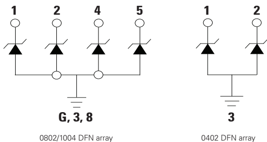
0802/1004 DFN array
