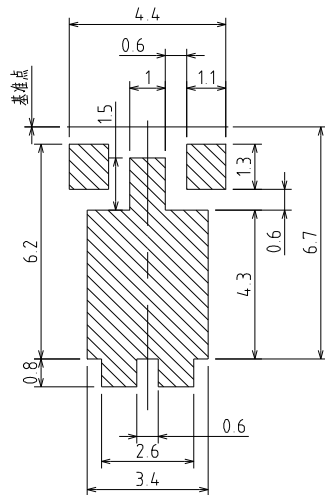
建议安装图
