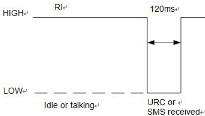
图表 24: 收到 URC 信息或者短信时 RI 时序
