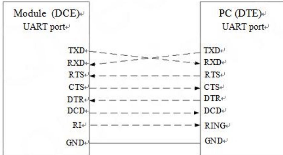
图表 10: 全功能串口连接方式示意图
