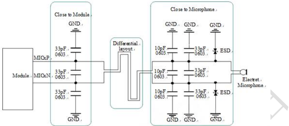
图表 17: AIN 麦克风通道接口电路
