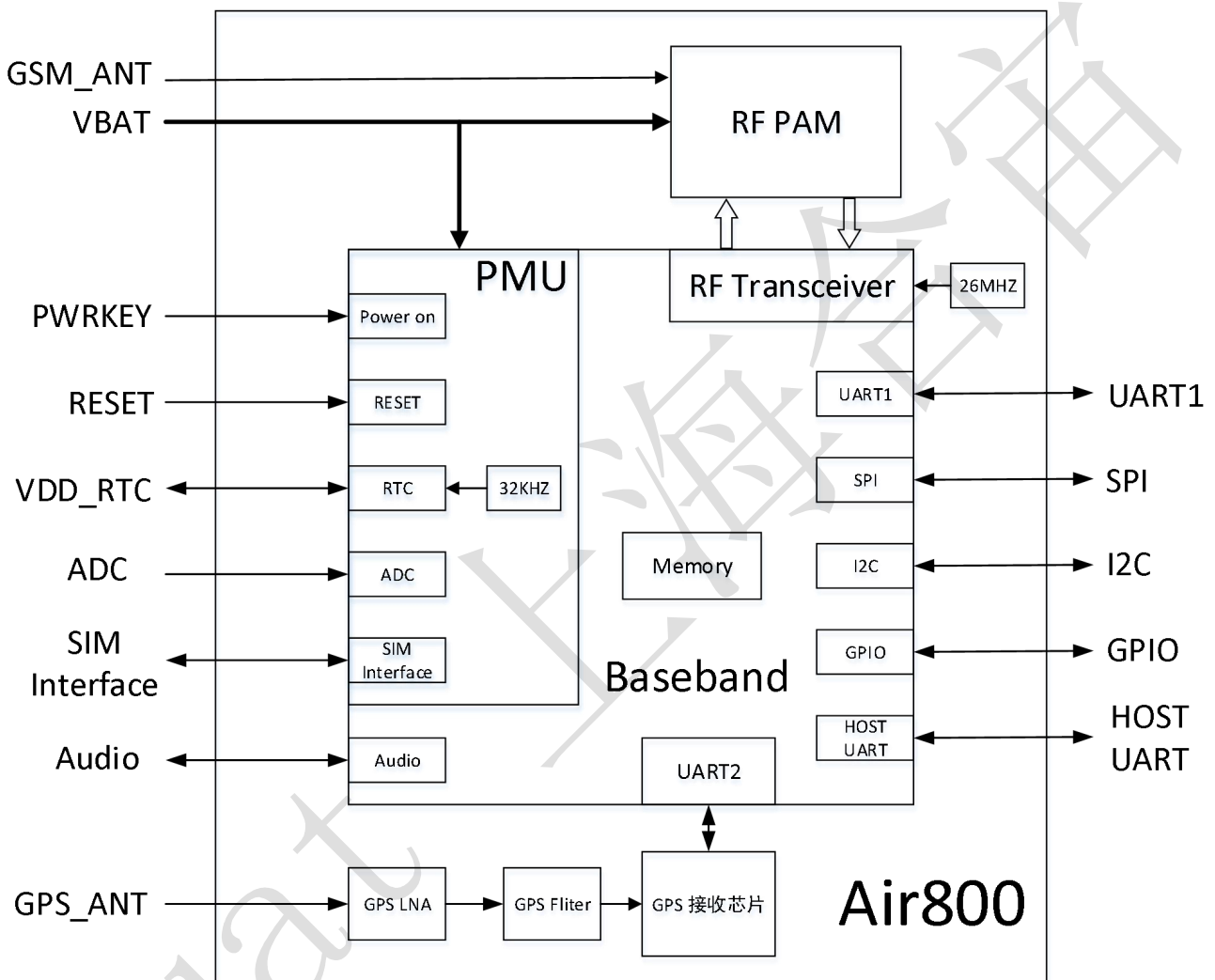
图表 1：功能框图
