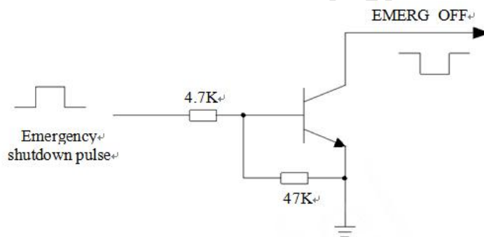
图表 8：开集驱动参考紧急关机电路
