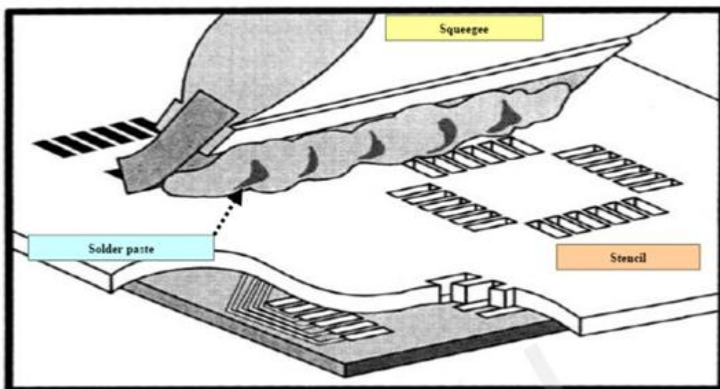
图表 32：印膏图
