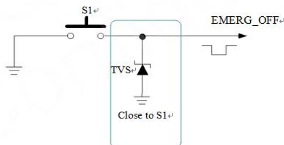
图表 9：按键紧急关机参考电路
