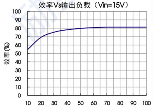
图3: 效率曲线图
