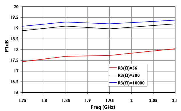
P1dB
