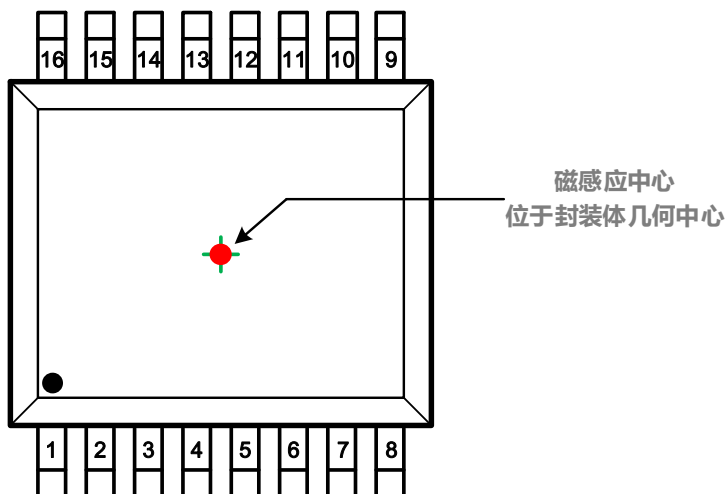
图-1: MT6835 TSSOP-16封装外观图
