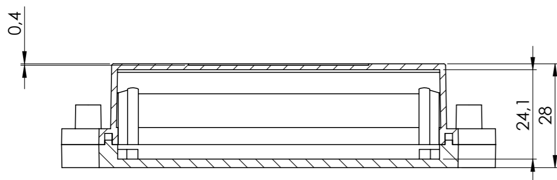
PRZEKRÓJ A-A
