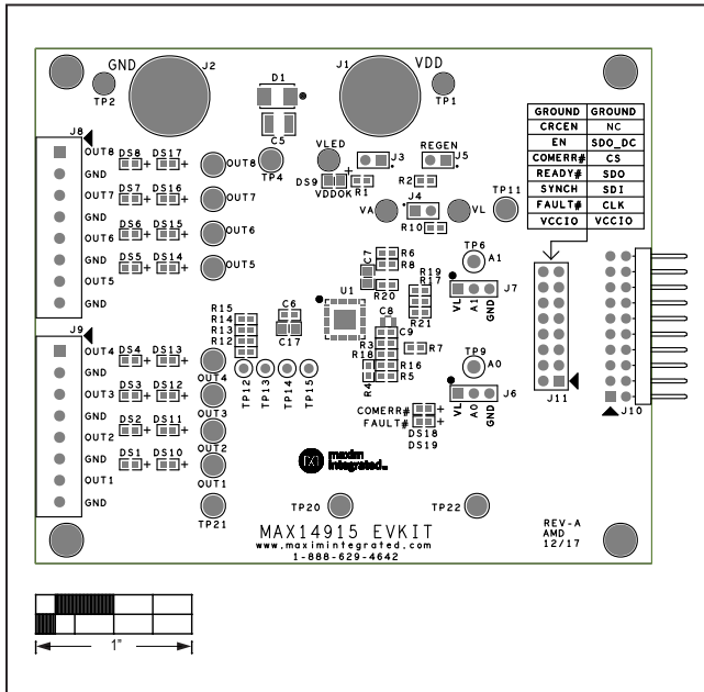
MAX14915 EV Kit—Silk Top
