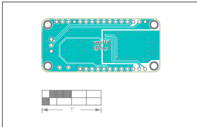
MAX86916 EV System—Top Layer
