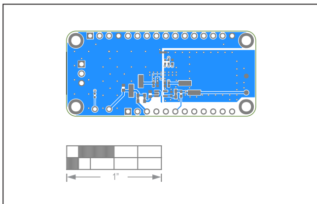
MAX86916 EV System—Bottom Layer
