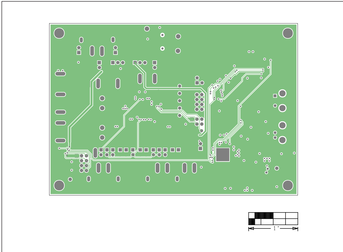
MAX98091 TQFN EV Kit PCB Layout—Internal Layer 3 SIG
