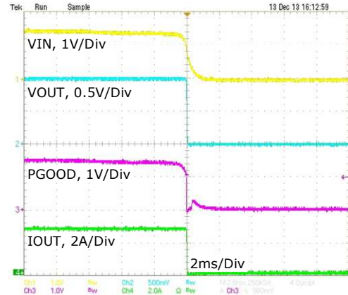
Fig. 11: Powerdown, IOUT=3A, 1.5VIN, 1VOUT
