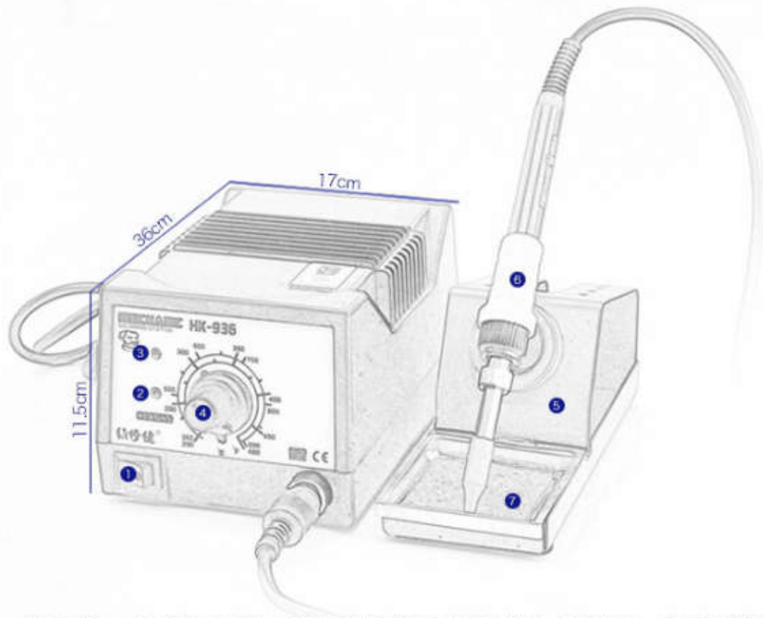
① 电源开关 ② 恒温指示灯 ③ 电源指示灯 ④ 温度调节钮 ⑤ 精制烙铁座 ⑥ 烙铁手柄 ⑦ 耐高温海绵
