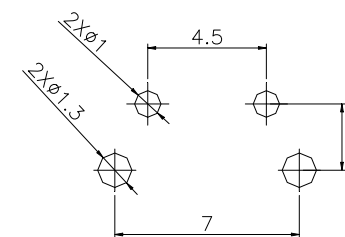
PCB. 焊接图
