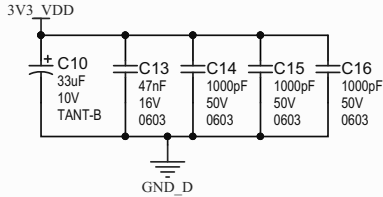
For VCCO_0
