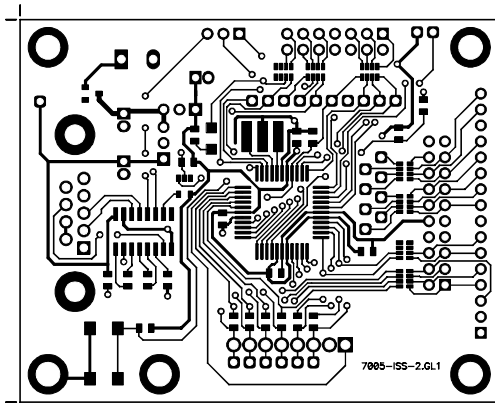
Figure 4 — Top Layer
