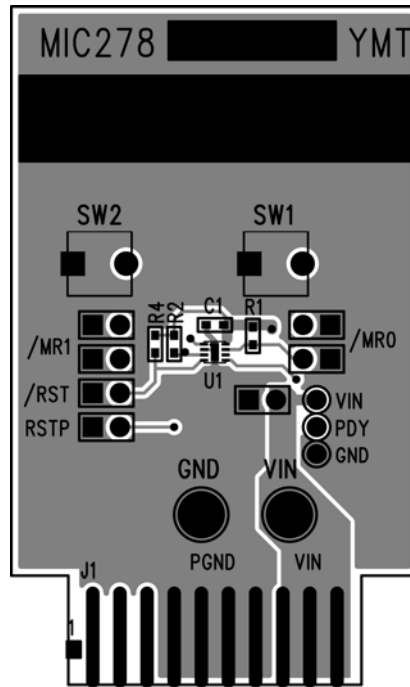
Copper Layer 1
