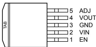
TO-263-5
