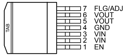
S-PAK-7
