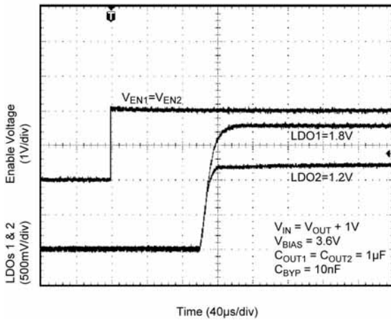
Enable Turn-On
